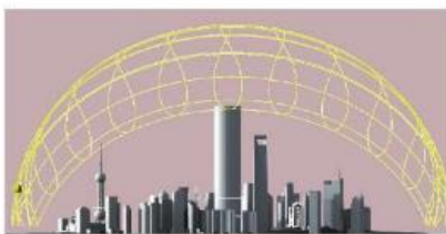
Pohyb slunce
